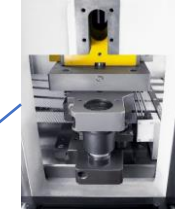
Druckgesteuertes Lamellenwerkzeug 3-6 Spuren 450-700 Breite
