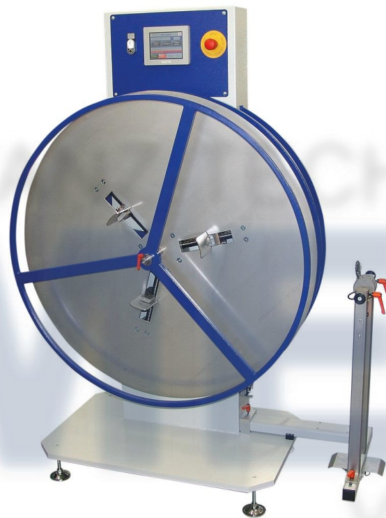
Vertikalwickler
